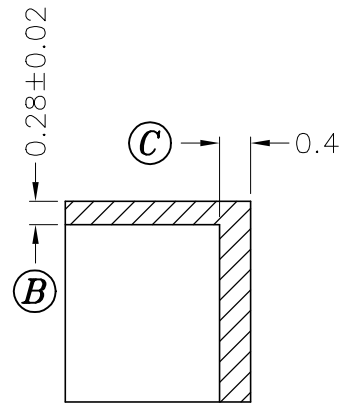
SEC. A-A
