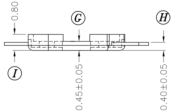
SEC.A-A
