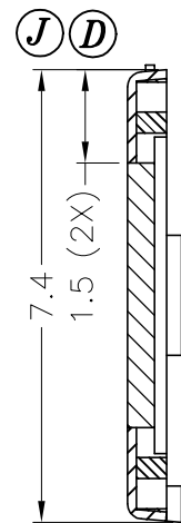
SEC. A-A
