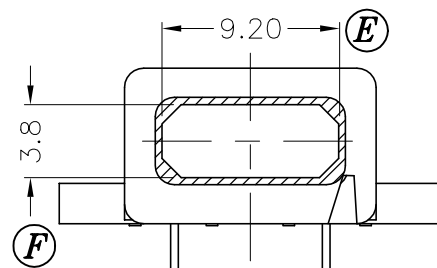
SEC. A-A
