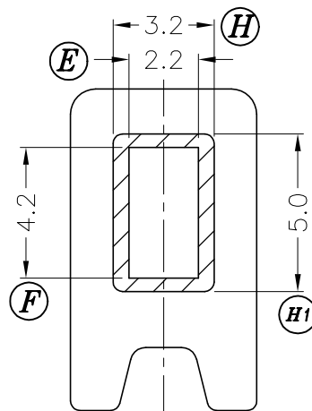
SEC.A-A
