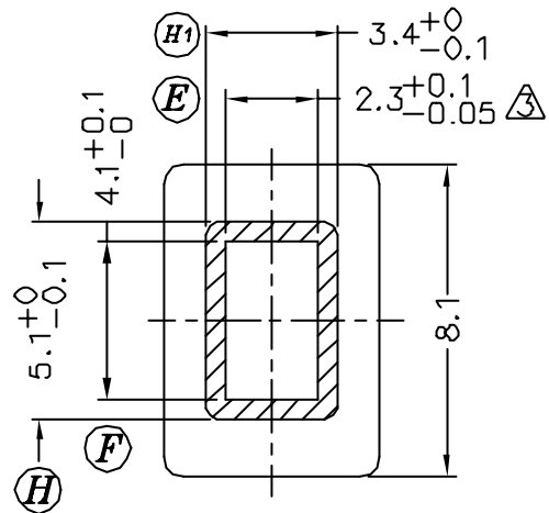
SEC.A-A
