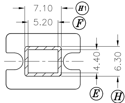
SEC. A-A
